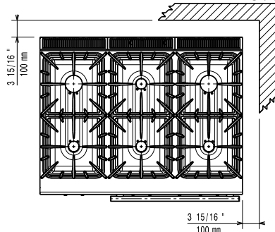
Boven aanzicht
